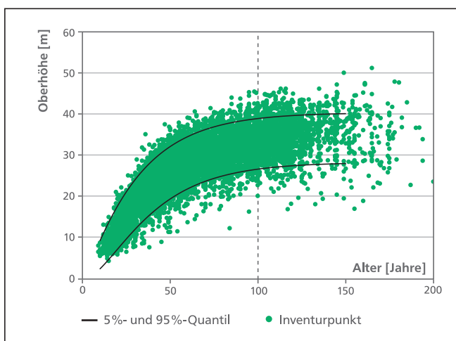
Leistungsdiagramm für Fichte
