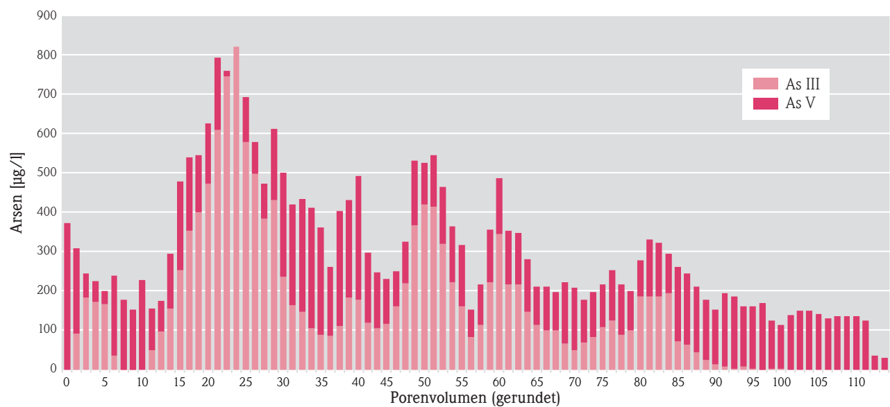
Abb. 2b und c: Oxische Versuche mit Substratbeaufschlagung.
