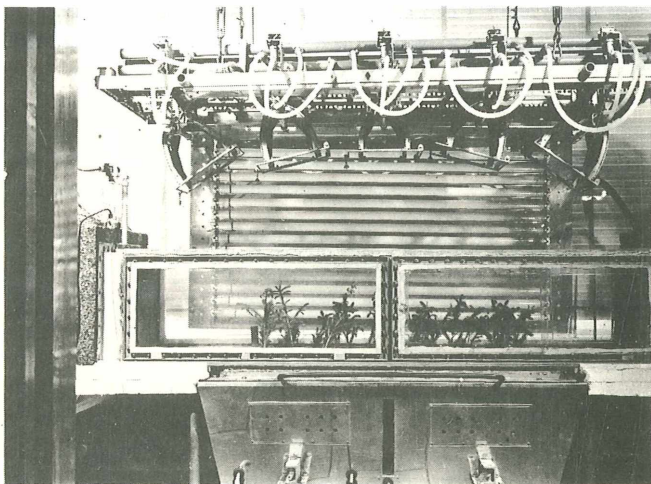
Abb. 9: Ansicht der Versuchsstrecke des Windkanals im Klimahaus auf dem Patscherkofel. Die Luft in der Versuchsstrecke wird durch einen Ventilator (im Bild nicht sichtbar) bewegt und beim Passieren einer Klimaanlage (im Keller des Hauses) auf die gewünschte Temperatur und Feuchtigkeit gebracht. Die Versuchspflanzen stehen auf einem Wagen und werden von unten in die Versuchsstrecke eingeführt. Darüber befindet sich die Beleuchtungsanlage, die aus Xenonlampen und Leuchtstoffröhren besteht.
