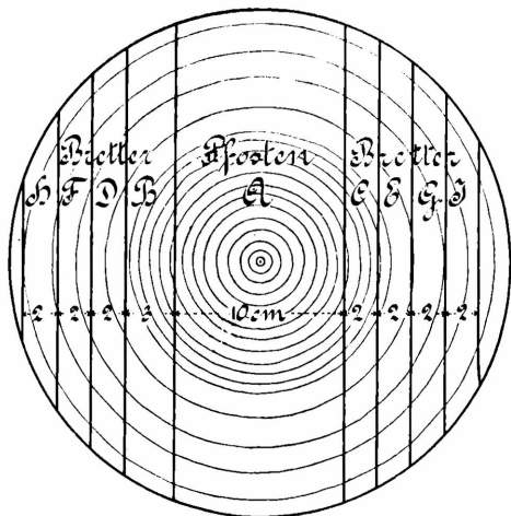
Fig. 8. Zerlegung des Rundholzes in Schnittholzsortimente.
