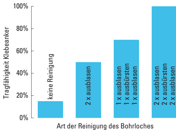
Abb. 2. Tragfähigkeit eines Klebeankers in Abhängigkeit der Reinigung des Bohrloches (nach Debrunner Acifer, 2015).
