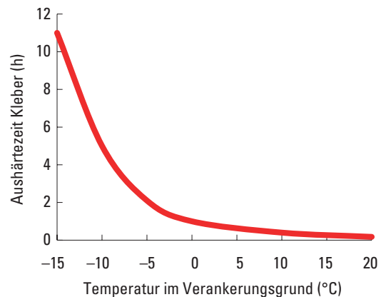
Abb. 3. Aushärtezeit eines Kunstharzklebers in Abhängigkeit der Temperatur des Verankerungsgrundes (nach Lang, 1979).
