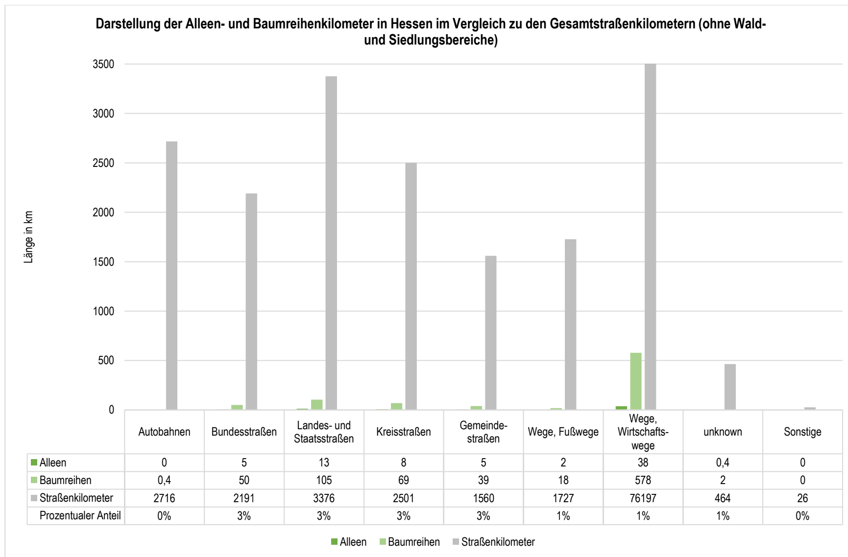
Abbildung 27: Grafische Darstellung der Alleen- und Baumreihenkilometer in Hessen im Vergleich zu den Gesamtstraßenkilometern
