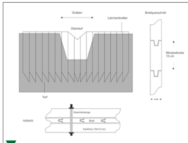
Schematische Darstellung eines Dammes für eine Wiedervernässung (Gert-Michael Steiner in: Aktiv für Moore, 2003).
